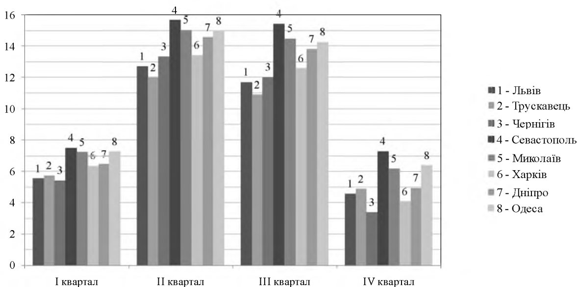
Рис. 4. Розраховане загальне поквартальне виробництво енергії на електростанції потужністю P_{nom, total} = 30 \text{ кВт}
