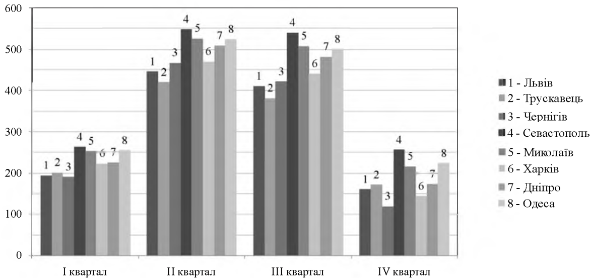
Рис. 3. Розраховане загальне поквартальне виробництво енергії на електростанції потужністю P_{nom, total} = 1 \text{ МВт}
